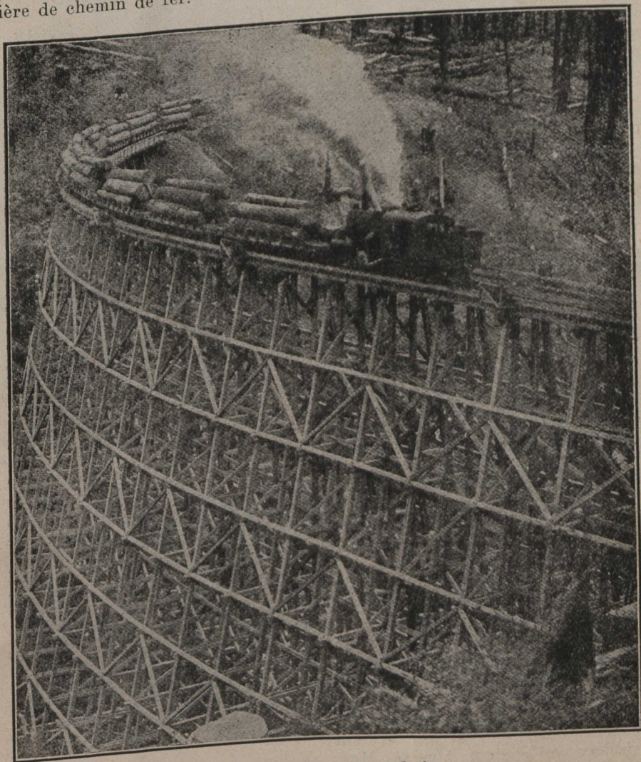
Pont sur tréteaux en bois.
