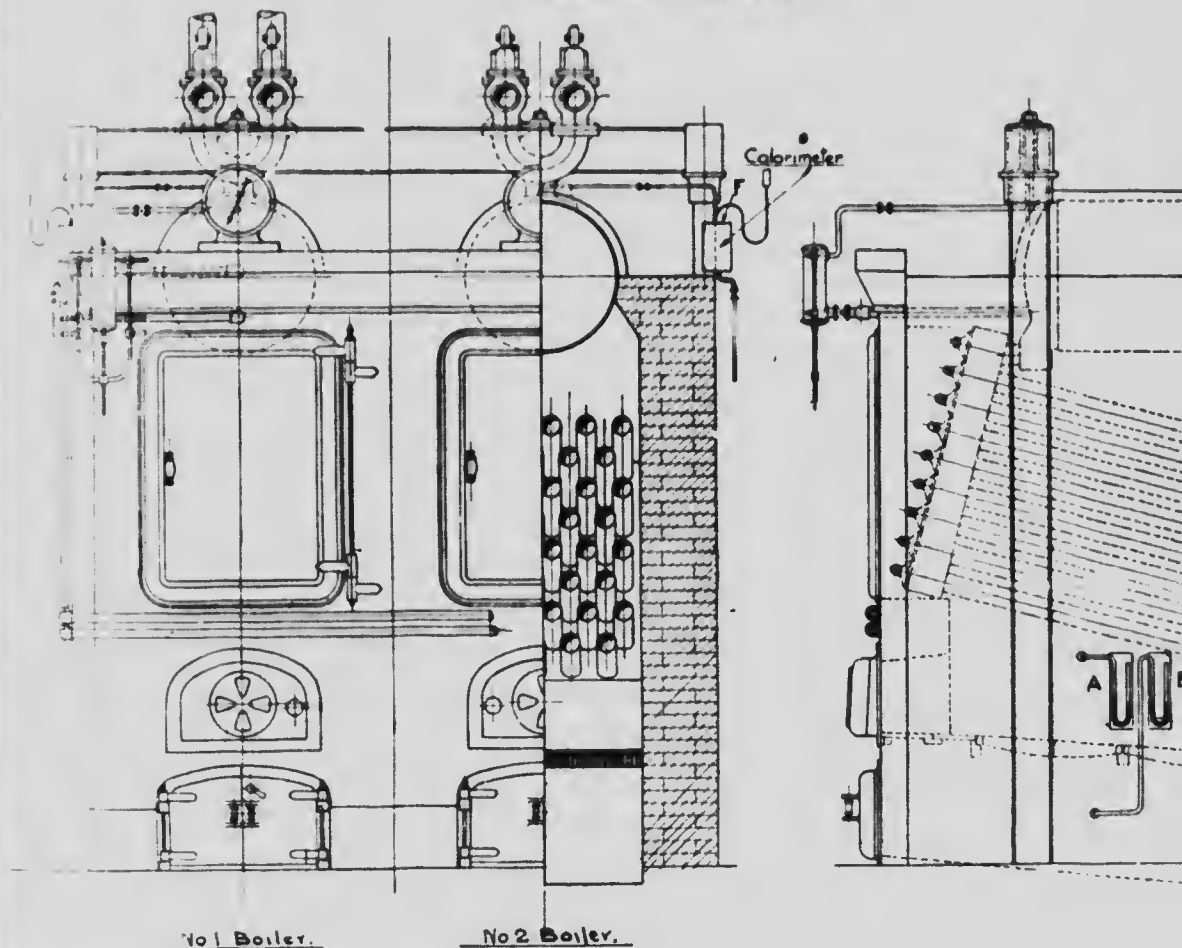
No 1 Boiler.
