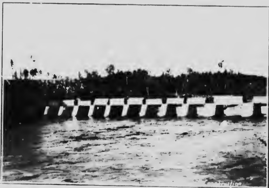
RIVER WISN. - BARRAGE DE LA COMPAGNIE CANADIENNE DU CANAL DU NIAGARA
