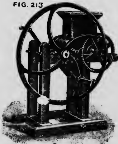
Désintégrateur à bras Dolberg pour mousse litière.
