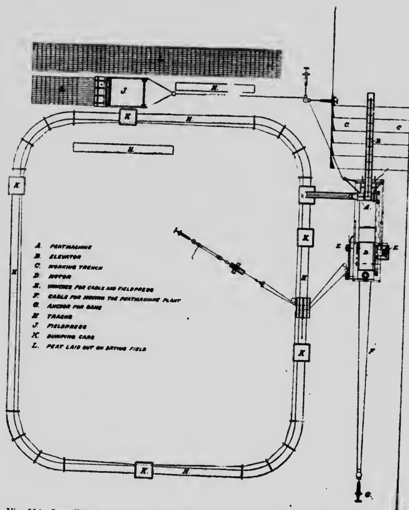
Fig. 114. Installation à tourbe Svedala d'Aurep avec transport par câble sur voie ronde, et presse portable.
