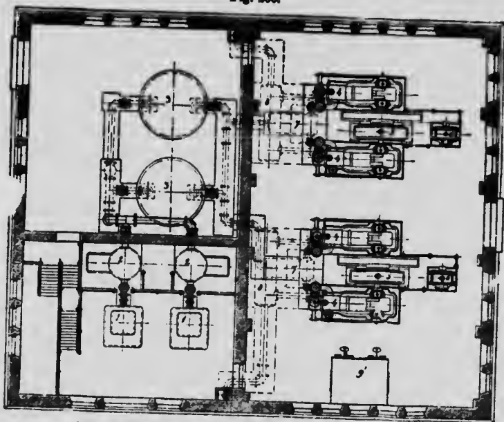
Machine de force motrice à gaz de tourbe à Skabersjö, Suède.
