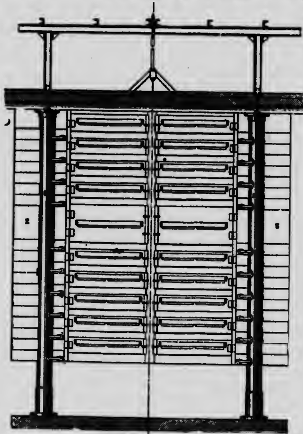
ig. 146. Séchoir à vapeur à plaques (vue latérale).
