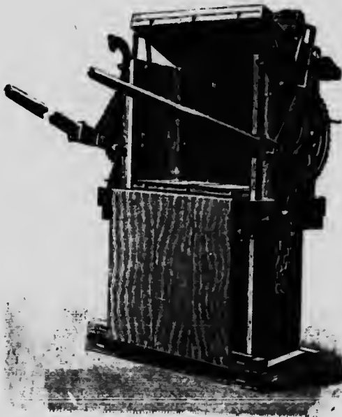
Fig. 224. Presse à mousses litière.
