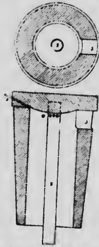
Fig. 172. Le four à carboniser la tourbe Hahneimain.
