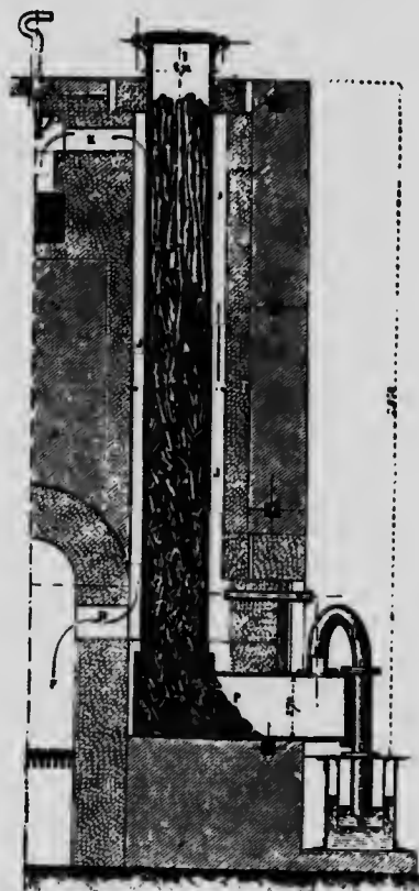
Fig. 211. Gazogène Riché.
