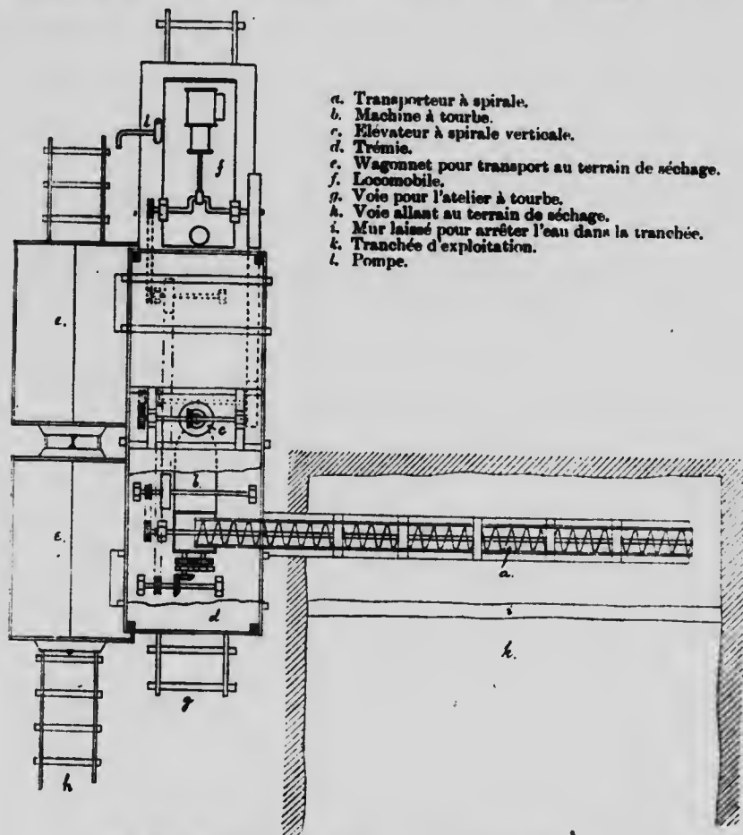
Fig. 39. Plan esquisse de l'usine à tourbe de Herning, Danemark.
