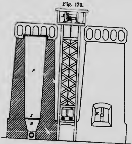
Le four à carboniser la tourbe Wagauman.
