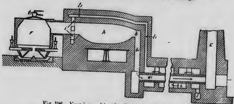
Fig. 196. Four à reverbère chauffé avec du gaz de gazogène.
