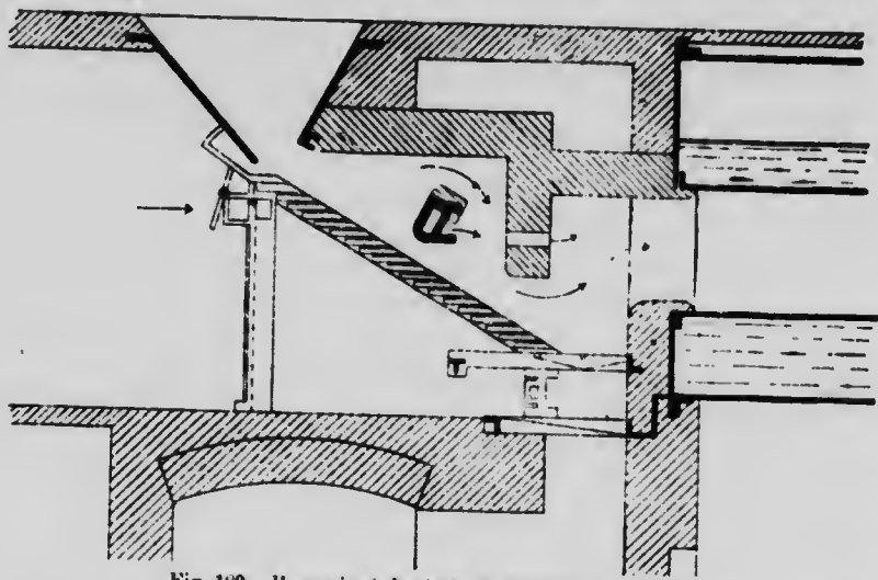
Fig. 189. Fournaise à demi-gaz de Keilmann et Volker.
