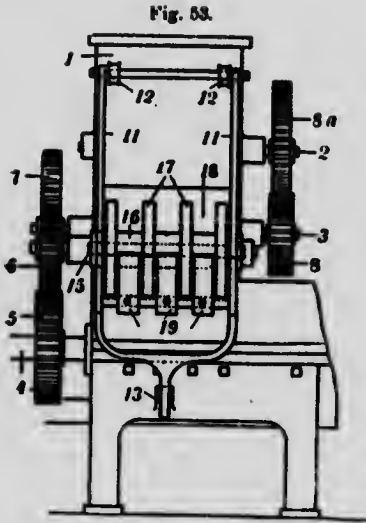
Machine à turbine Schlickeysen N° 3.
