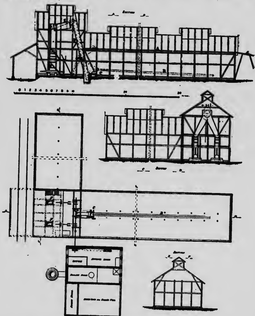
Fig. 228. Usine à tourbe litière avec deux presses.
