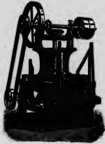
Fig. 220. Moulin à poussier de tourbe de A. Heinen.
