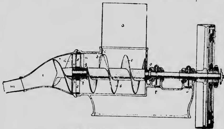
Fig. 88. Machine à tourbe Svedala N° 2.
