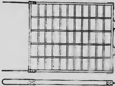
Fig. 37. Moules à tourbe employée à Okaer.
