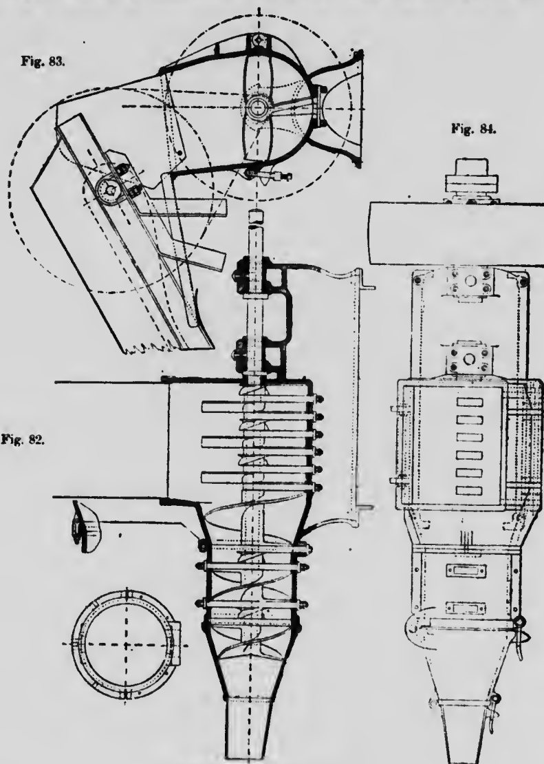
Machine à tourbe de Aurep, No. 1B.
