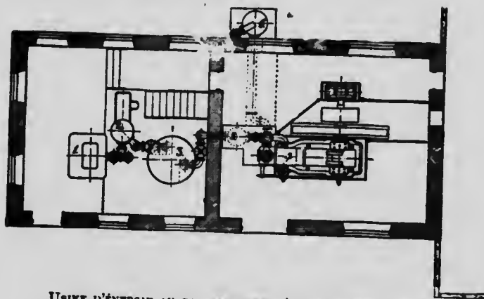
USINE D'ÉNERGIE AU GAZ DE TOURBE, À BURÅNGSBERG, SUÈDE
