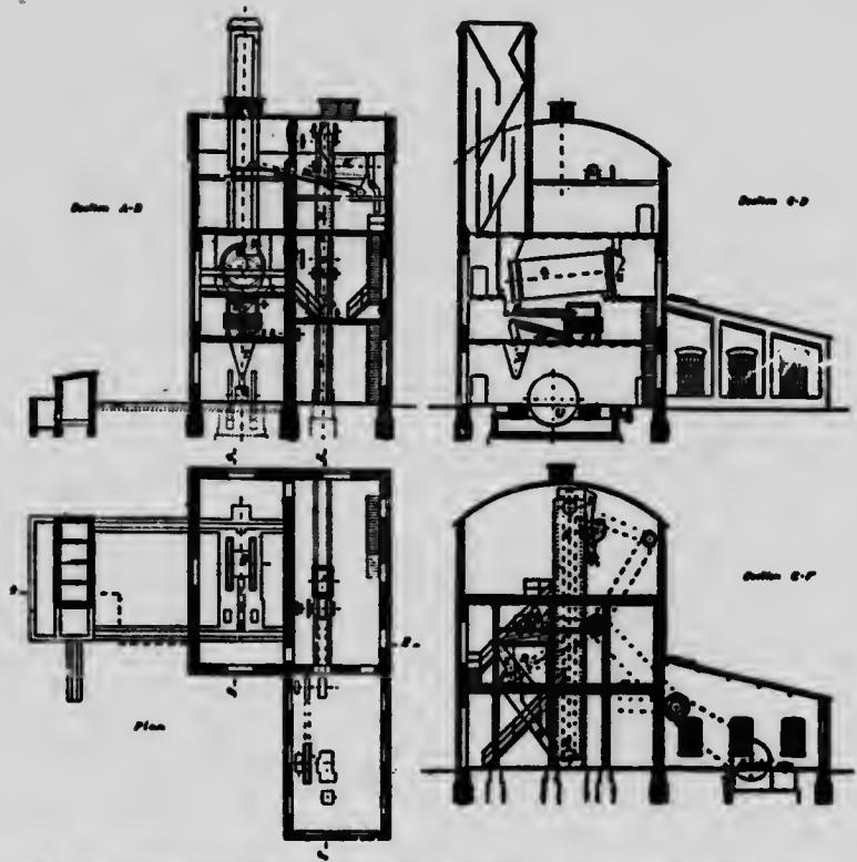
Fig. 163. Installation pour fabrication de briquettes de tourbe avec un séchoir Schulz.
