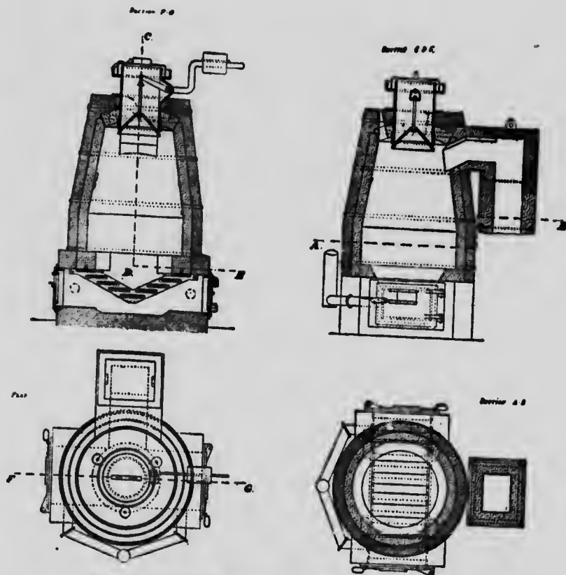
Fig. 193. Gazogène à tourbe aux Usines de fer Kollawa, Suède.
