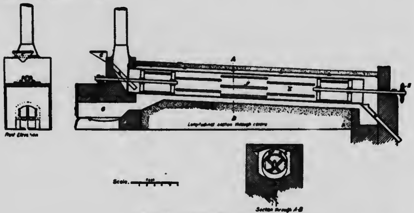
Fig. 168. Le séchoir "Dobson".
