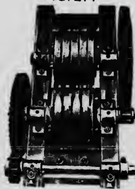
Désintégrateur à bras Dolberg pour mousse litière.
