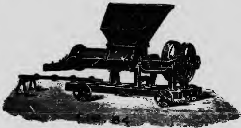
Fig. 64. Machine à tourbe Dolberg, N° 1b, (extérieur).
