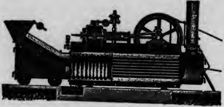
Fig. 185. Locomobile avec grille à échelons de H. Lanz, Mannheim, Allemagne.
