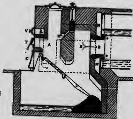
Fournaise à demi-gaz de C. Reich.
