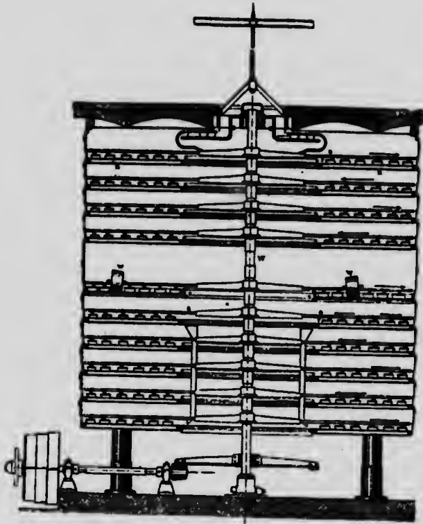
Fig. 147. Séchoir à vapeur à plaques (coupe).
