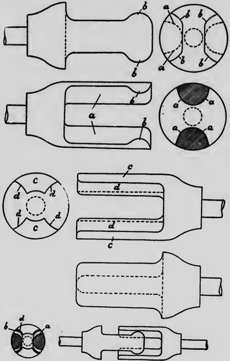
Fig. 120. Accouplage du Convoyeur à tourbe Kärner.
