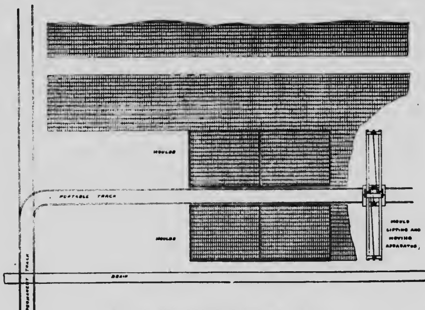
Fig. 40 Terrain de séchage à Herning, Danemark.
