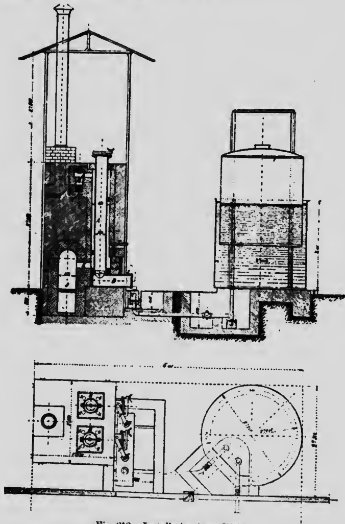
Fig. 212. Installation à gaz Riché.
