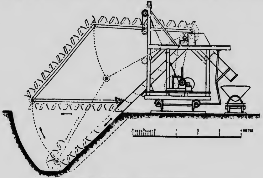
Fig. 58. Excavateur à tourbe Schlikeysen.
