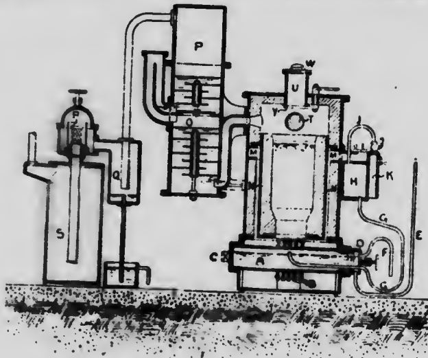
Fig. 200. Outillage à gazogène Bénier pour anthracite et coke.
