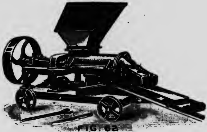
Fig. 62. Machine à tourbe Dolberg, N° 1a, (extérieur).
