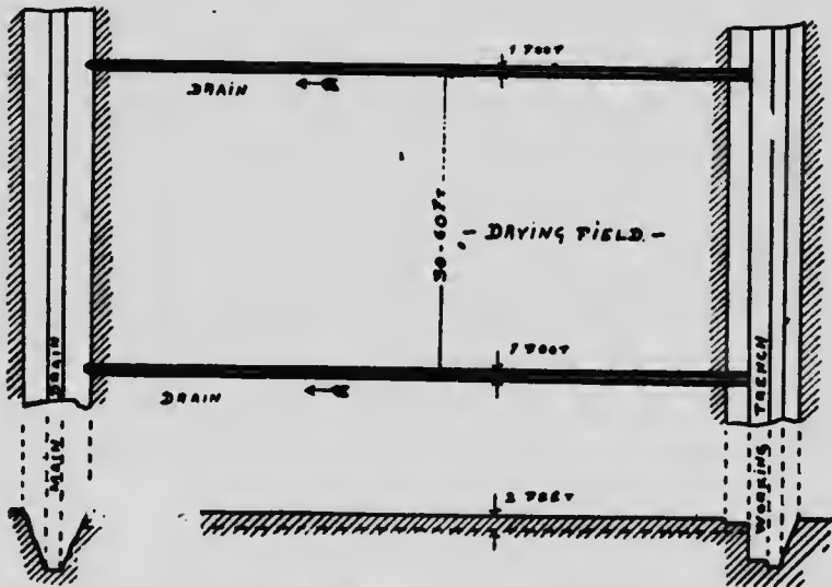
Fig. 2. Méthode de drainage.
