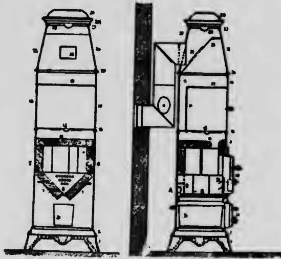
Fig. 182. Poêle à tourbe de Reck.
