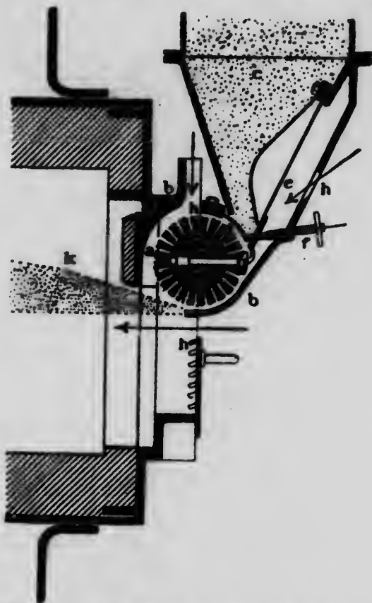
Fig. 192. Appareil pour souffler la poudre. (Schwarzkopf).
