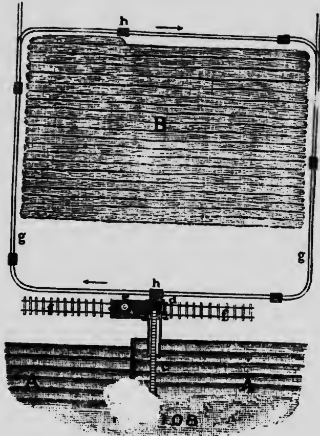
Fig. 108. Transport et étente pour séchage avec voie ronde. (B. mottes de tourbe étendues).
