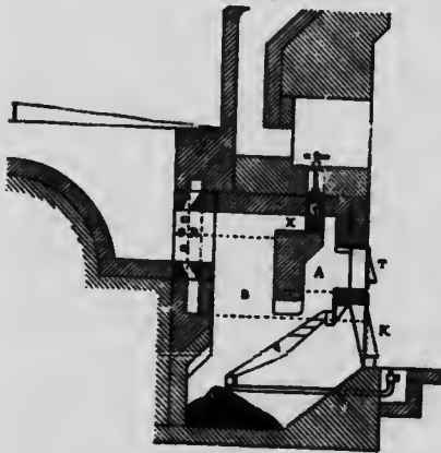
Fournaise à demi-gaz de C. Reich.
