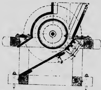
Fig. 219. Désintégrateur à pouvoir moteur de Aljorn Anderson's pour mousse litière.
