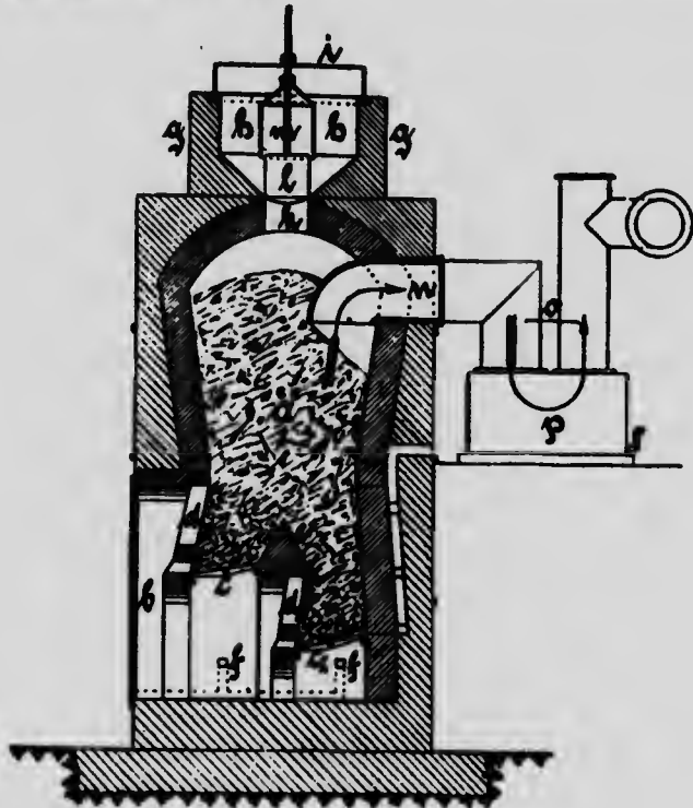
Fig. 210. Gazogène à tourbe de Ziegler.
