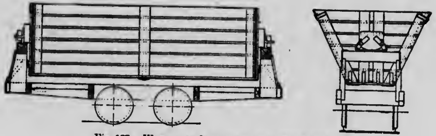
Fig. 127. Wagon pour le transport de la tourbe séchée.
