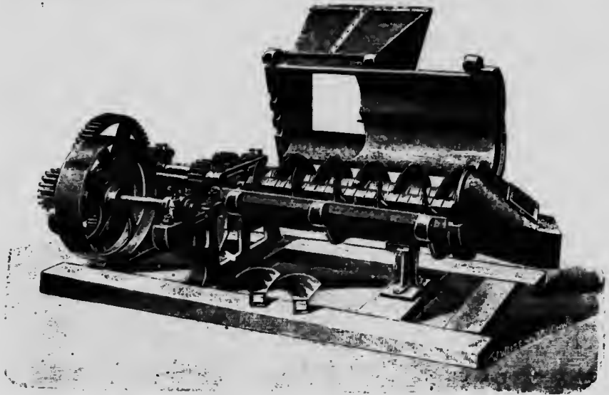
Fig. 72. Machine à tourbe N° T1 et T2 du type Dalberg, par A. Heinen.
