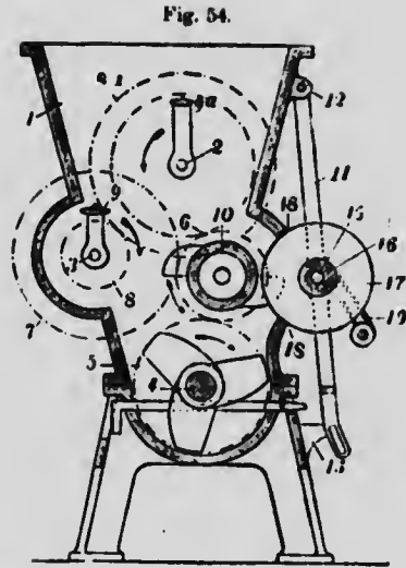
Machine à turbine Schlickeysen N° 3.
