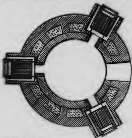
Fig. 107. Four à chaux avec demi chauffe à gaz.
