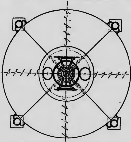
Fig. 148. Séchoir à vapeur à plaques (plan).
