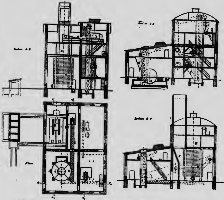
Fig. 162. Installation pour fabrication de briquettes de tourbe avec une presse et un séchoir à plaques à vapeur.
