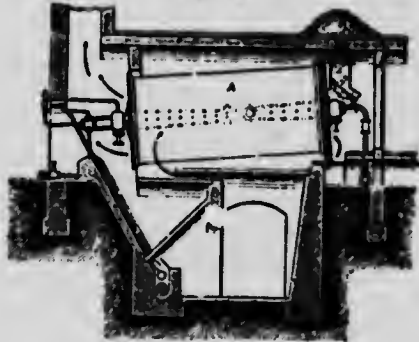
Séchoir Schulz.
