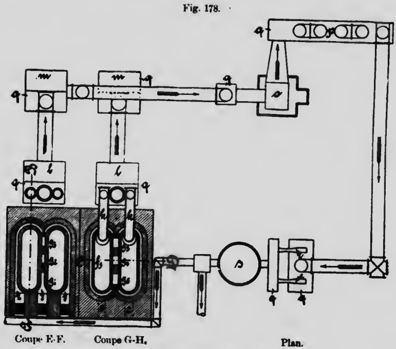
Conduites à carboniser la tour de Ziegler.
