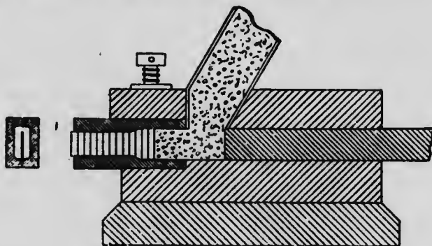
Fig. 155. Coupe de la presse à briquettes.
