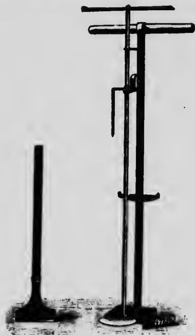
Fig. 27. Petite machine à couper, R. Dolberg.
