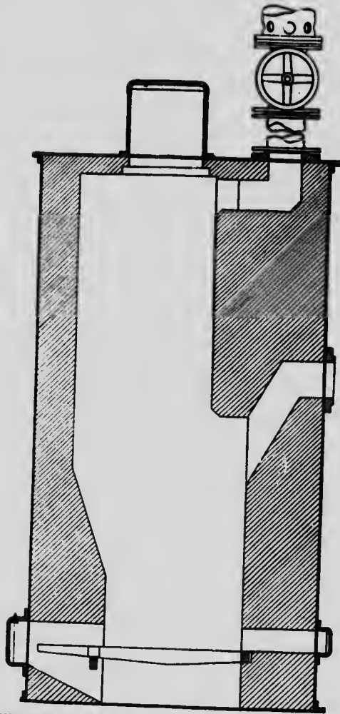
Fig. 203. Gazogène à briquettes de lignite de Korting.
