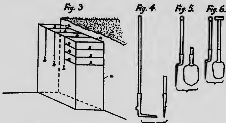
Méthode pour couper la tourbe et outils employés à Sparker, Danemark.
