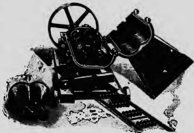
Fig. 67. Machine à tourbe Dolberg, N° 1e (intérieur).
