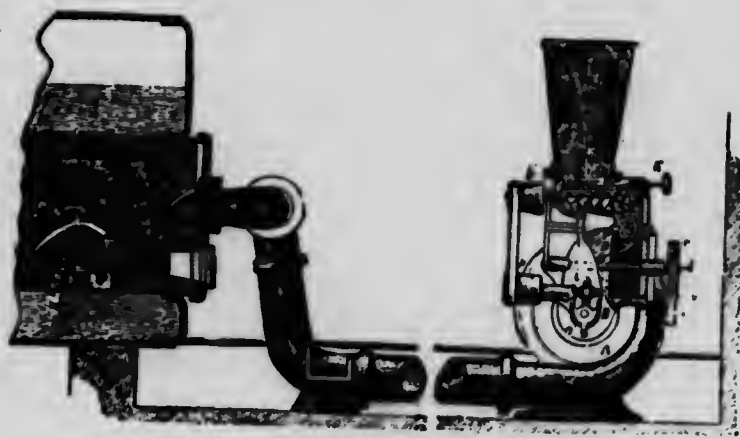
Fig. 190. Appareil F. de camp pour brûler poudre de tourbe.
