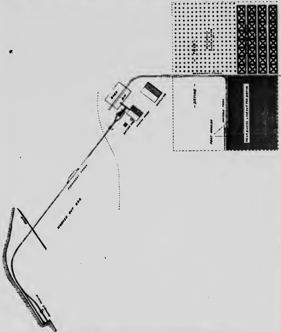
Fig. 34. Esquisse du plan de l'atelier à tourbe de Økaer, Danemark.
