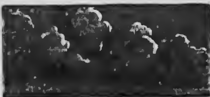
Cumulus
