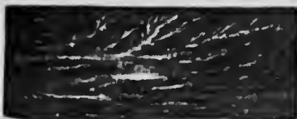
Cirrus
