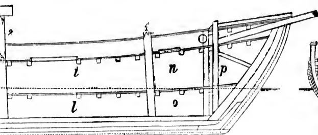
Længdesnit.
