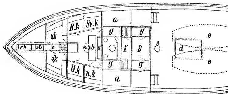
Fig. 2. Plantegning.
