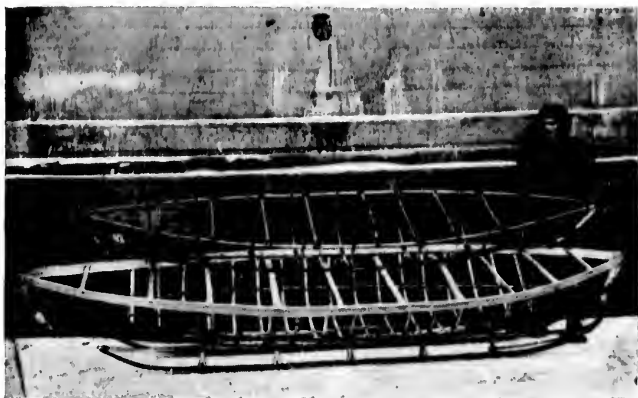
Skeletter af en enkeltkajak, af bambus, og en tomands-kajak, på en kjælke. Fotografi.
