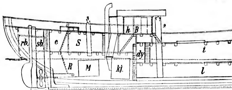
Fig. 1. Længdesnit.
