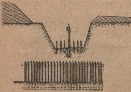
Coupe d'un fossé avec palissade protégeant les tranchées.
