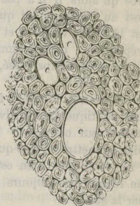
Fig. 3.—Cellulose.
