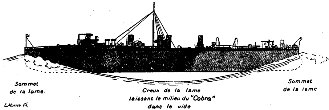
Croquis montrant comment a pu se produire la rupture du torpilleur Cobra en son milieu
