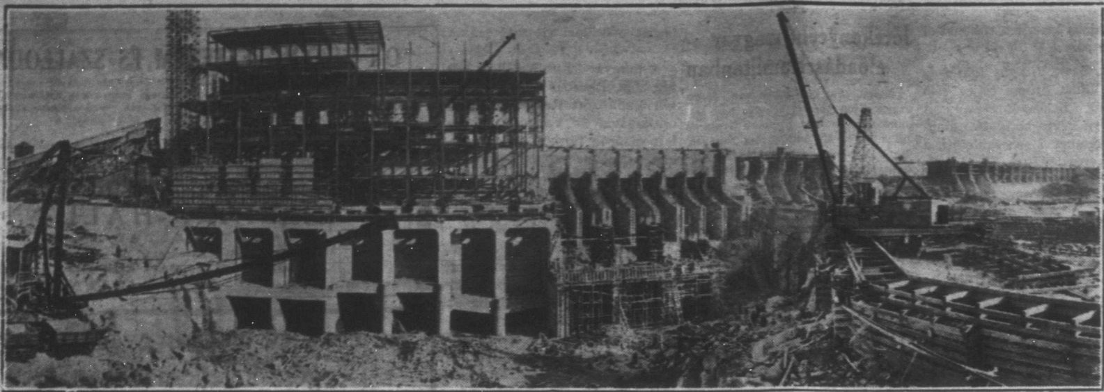
A Winnipeg folyó vízijerének felhasználása céljából a Seven Sisters zuhatagnál már teljesen elkészült az új villamos áramfejlesztőtelep váza, amint azt fenti képünkön is láthatjuk olvasóink. A tervező mérnökök kiemelt szerepet szenteltek a dinamókat is, melyek egyelőre 42 ezer lóerőt foglalkoztatnak tudni kifejteni. Néhány éven belül azonban a telep energiakapacitását 225 ezer lóerőre szeretnék emelni, hogy Manitoba déli részét egészen elláthassák villamos árammal. A huszonötmillió dollár költséggel épített turbinaház és duzzasztógát munkálatainak több honfitársunk még ma is dolgozik, noha az eddig alkalmazott 1,200 munkás egy részét már elbocsátották.
