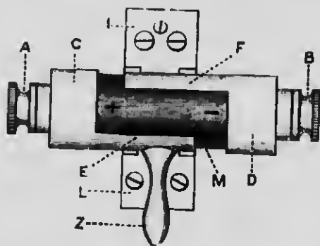
FIG. 26.—COMMUTATOR OF RUHKORFF.
