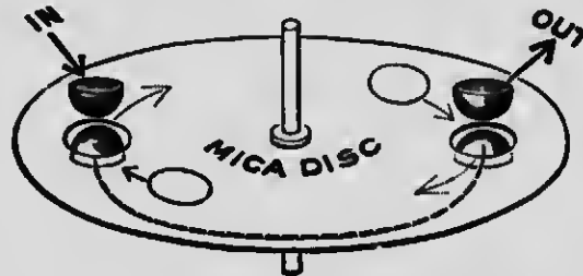
FIG. 113.—REVOLVING DISC RECTIFIER.
