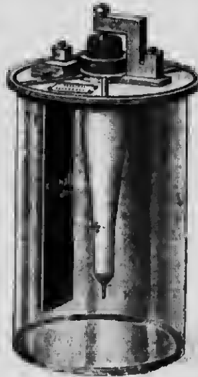
FIG. 105.—WEHNELT INTERRUPTER.
