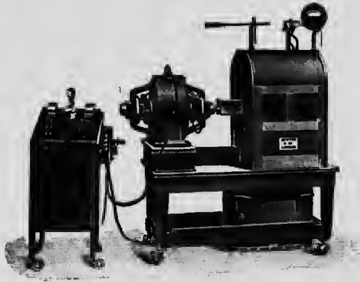
FIG. 110.—THE SNOOK APPARATUS.
