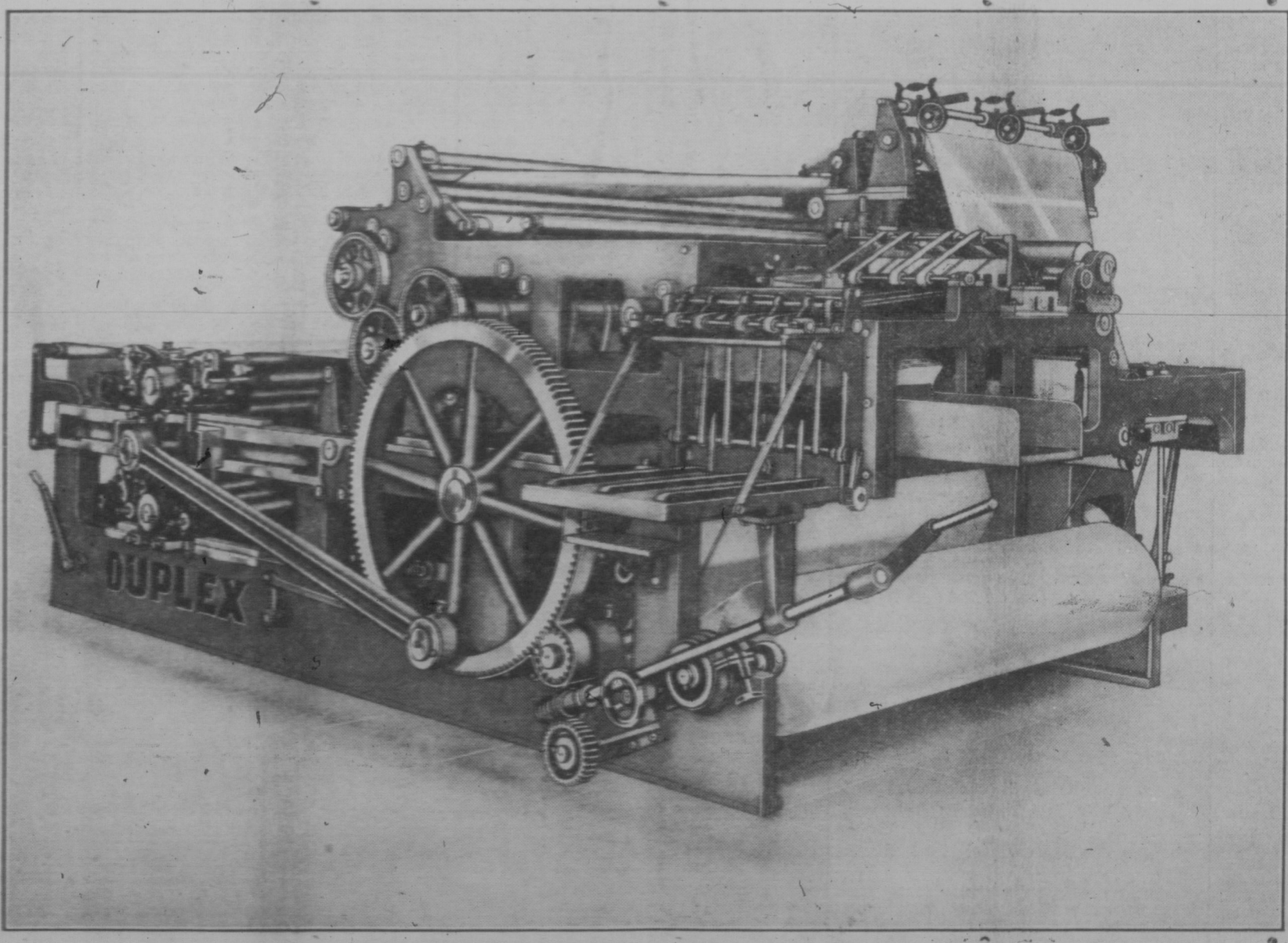
Das neue Modell der E Duplex-Pressen, auf welcher „Der Courier“ jetzt gedruckt wird.
