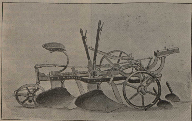
Charrue canadienne dite "Sulky" pour terre pesante. Capacité : 16 à 20 pes de large, 4 à 8 pes de profondeur.
