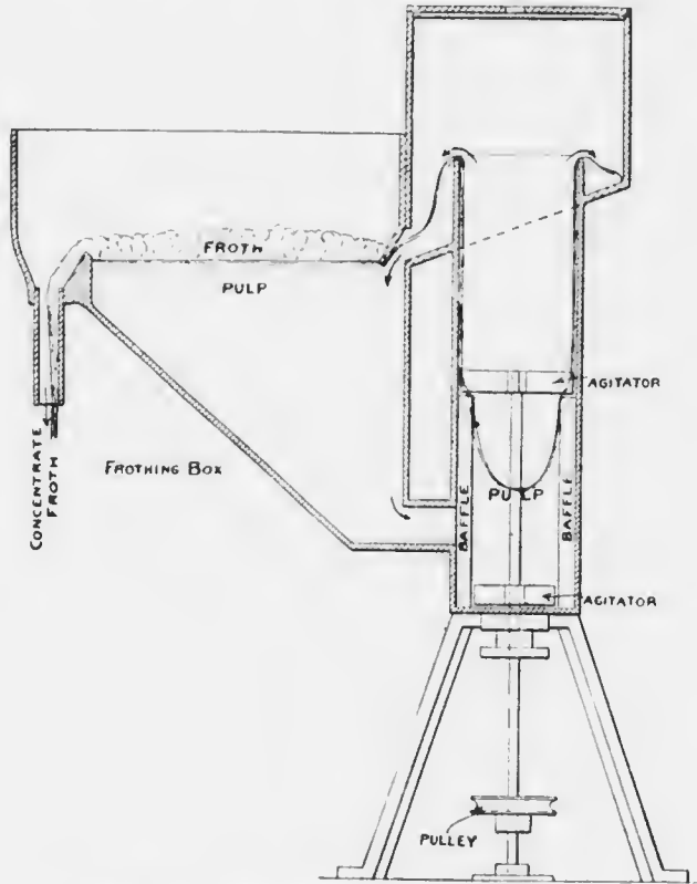
FIG. 27. THE JANNEY FLOTATION MACHINE.
