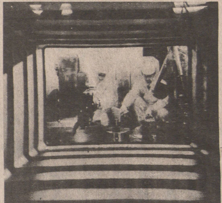
身穿氣衣的工作人員在熱室內進行放射性計量檢查和設備維修工作。
