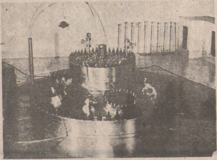
我國自行設計建造的第一座高通量反應堆。
