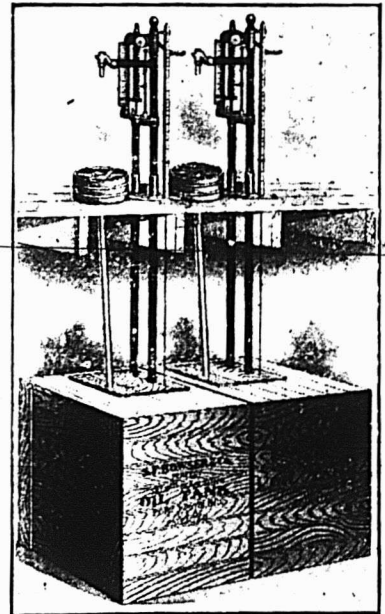
Gravure No. 35 Appareil de cave pour deux sortes d'huile.
