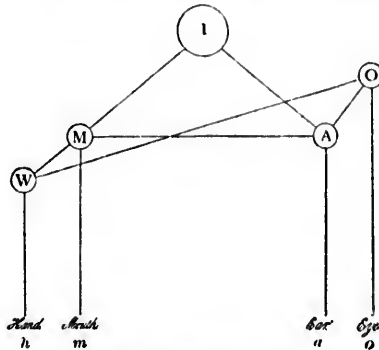
FIG. 5.—Lichtheim's schema.
