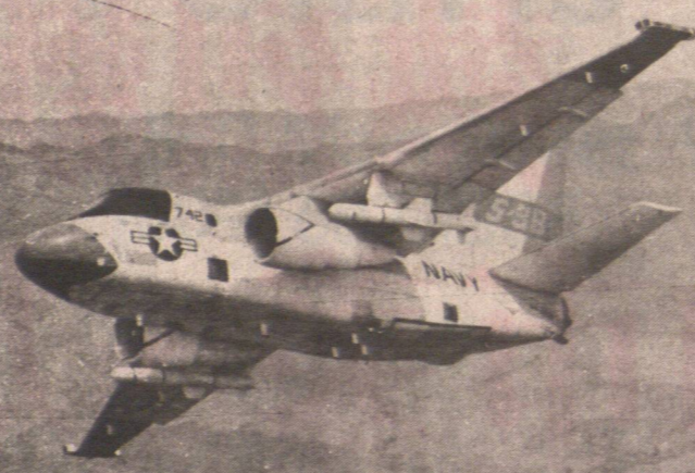
維京式飛機最近試驗，展示了它的超卓性能。由圖中可見，魚叉飛彈安裝在機翼下，電子支援測量(ESM)系統則設在機尾。
