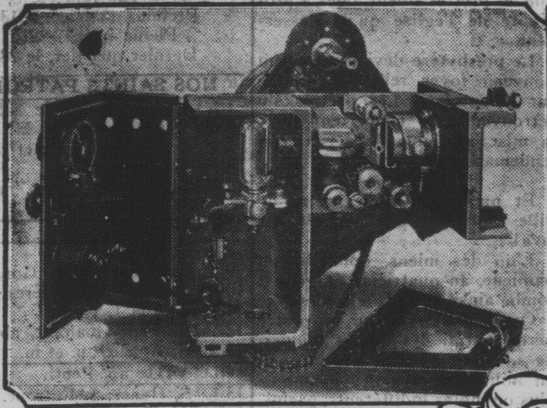
1. L'intermédiaire.—L'œil des pellicules sonores.—La lampe projette un rayon de lumière, sur une cellule photo-électrique, dans une proportion exacte aux variations des courants que l'on voit sur le circuit de la pellicule, tout en variant le courant dans les circuits de projection orale qui reproduisent les sons, par les haut-parleurs.
