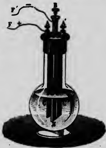
Fig. 212.—Pile de Grenet.
