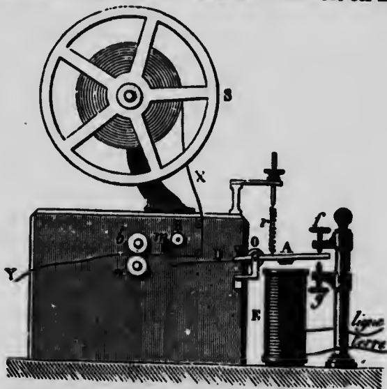
Fig. 220. — Récepteur Morse.
