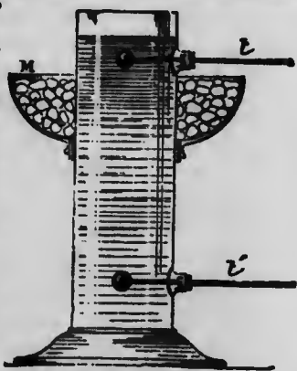
Fig. 187. — Maximum de densité de l'eau.
