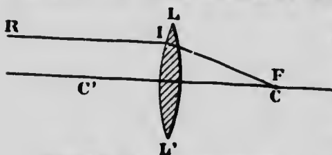
Fig. 193. — Lentille convergente.
