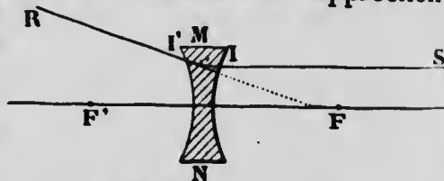
Fig. 194. — Lentille divergente.
