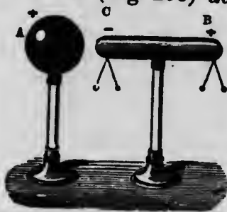
Fig. 206.—Influence électrique. charge de nom contraire à celle de la source qui a produit l'influence.
