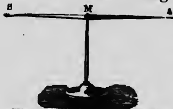
Fig. 199. — Aiguille aimantée.
