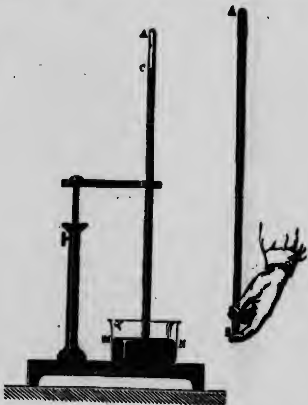
Fig. 171.—Expérience de Torricelli
