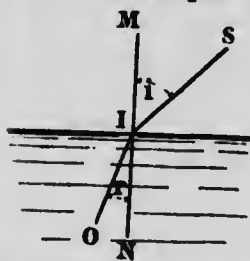
Fig. 191.—Réfraction de la lumière.
