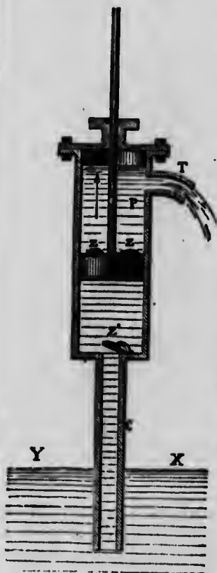
Fig. 176.—Pompe aspirante.
