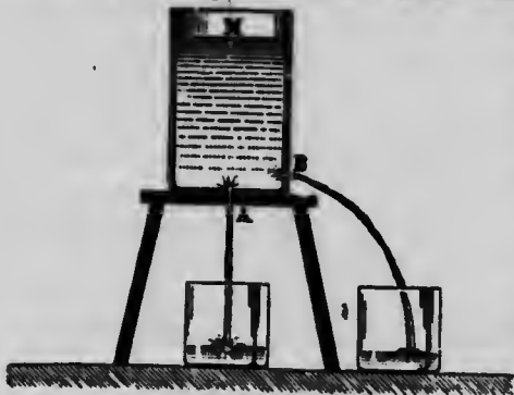
Fig. 163. — Pression latérale exercée par les liquides.
