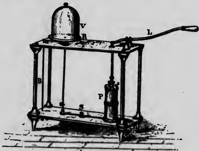
Fig. 174.—Machine pneumatique.
