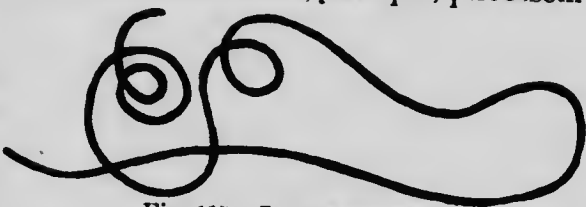
Fig. 115.—Le Dragonneau.
