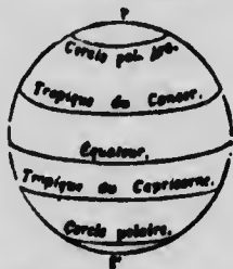
Fig. 227. — Cercles polaires et tropiques.
