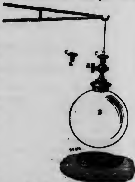
Fig. 168. — Poids des gaz.
