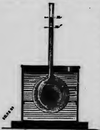
Fig. 186. — Dilatation des liquides.
