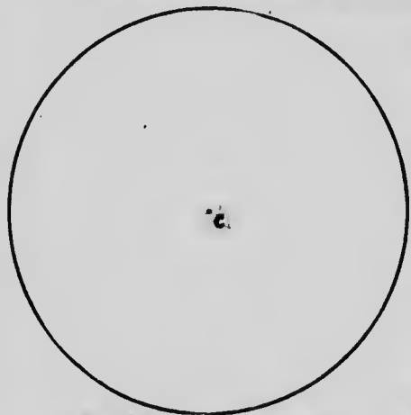
Fig. 224.—Circonférence.
