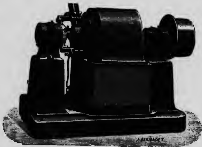
Fig. 215.—Machine dynamo-électrique.
