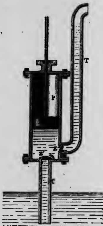
Fig. 177.—Pompe aspirante et foulante.
