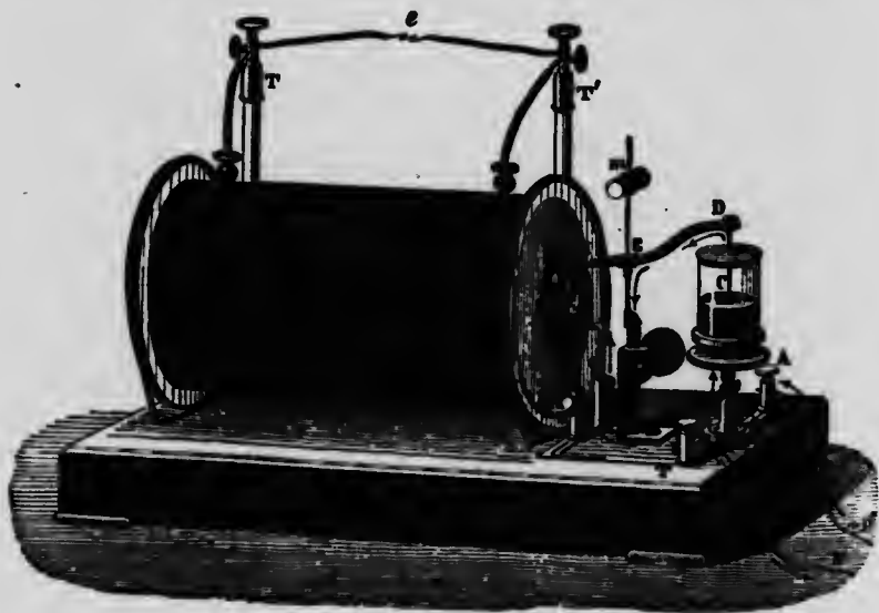
Fig. 214.—Bobine de Ruhmkorff.
