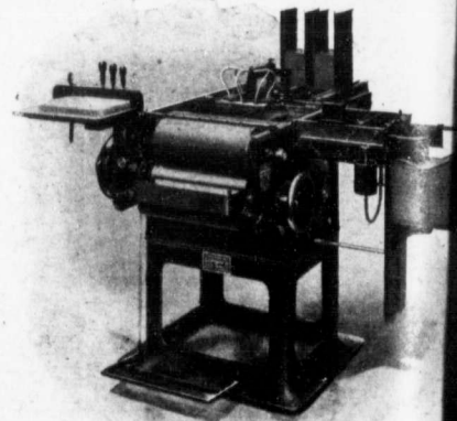
MACHINE A RELIER Pouvant fabriquer 400 couvertures de livres en une heure.
