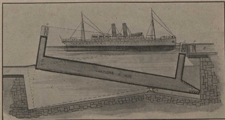
L'écluse-bascule placée à haut niveau
