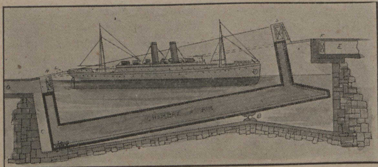
L'écluse-bascule à bas niveau
