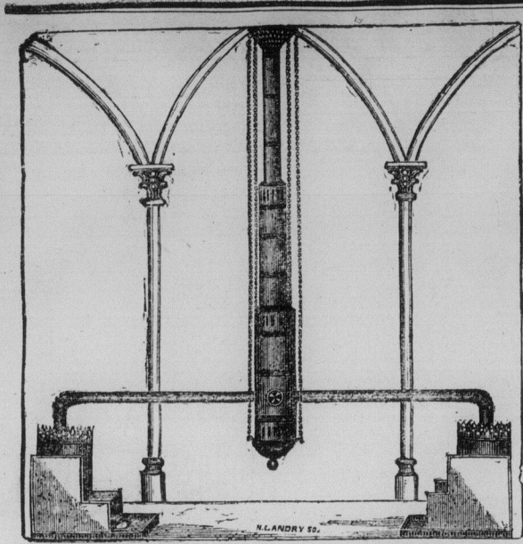
Système nouveau et amélioré pour chauffer les Eglises
