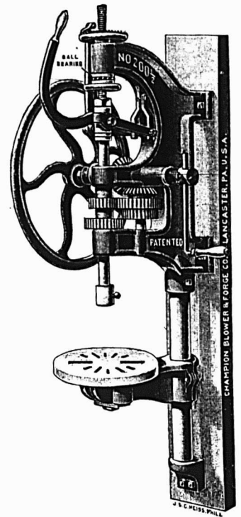
No 200 1/2 — Forerie Champion à colonne, alimentation automatique et alimentation à levier, Coussinet à Billes; Trous forgés jusqu'à 1 1/2 pce; et au centre d'un cercle de 18 pouces; poids, 225 lbs.
