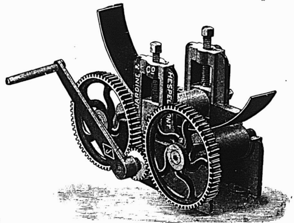
No 2 — Capacité, 4 pces de largeur ou 2 x 1/2 pces Poids, 120 lbs.
