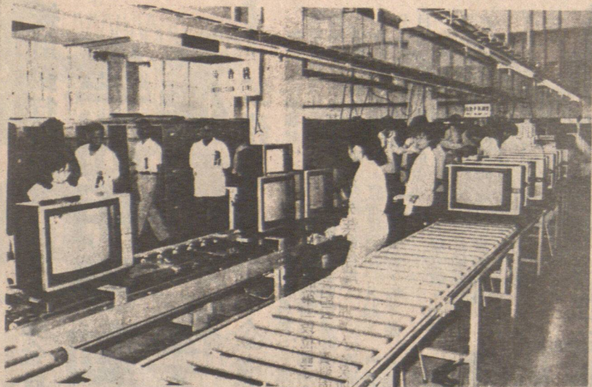
◀ 深圳華利電子有限公司新引進的日本「索尼」彩色電視機生產線已投產，年產十萬台。 ◀ 噸千二萬一產年，備設先進進口國外從廠材製鋁箔等。開車延壓為圖
