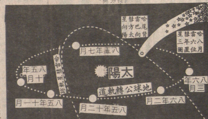
哈雷彗星明年回歸軌跡圖
