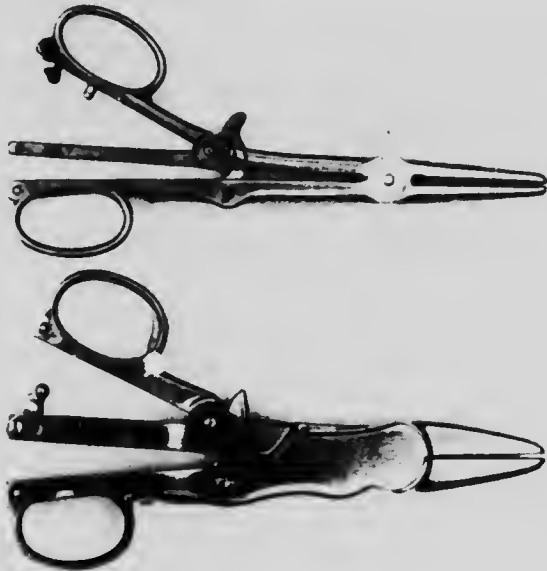
FIG. 125. AUTHOR'S ÉCRASEUR: PRIMARY AND FINAL MODELS
