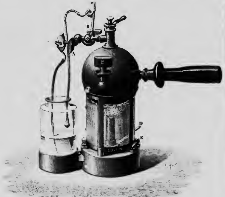
FIG. 312. —PULVERIZER OF J. LUCAS-CHAMPONNIÈRE.
