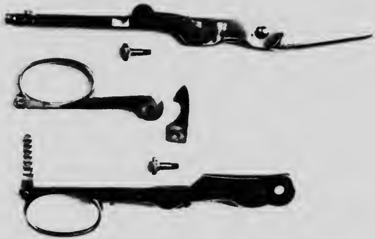
FIG. 112. ALMOND'S ÉCRASEUR: SECOND MODEL.
