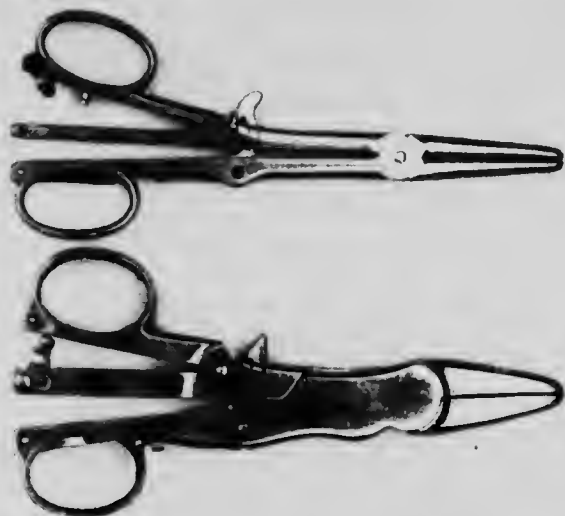
FIG. 127. ALLDOR'S ÉRASEUR: ORIGINAL AND FINAL MODELS.
