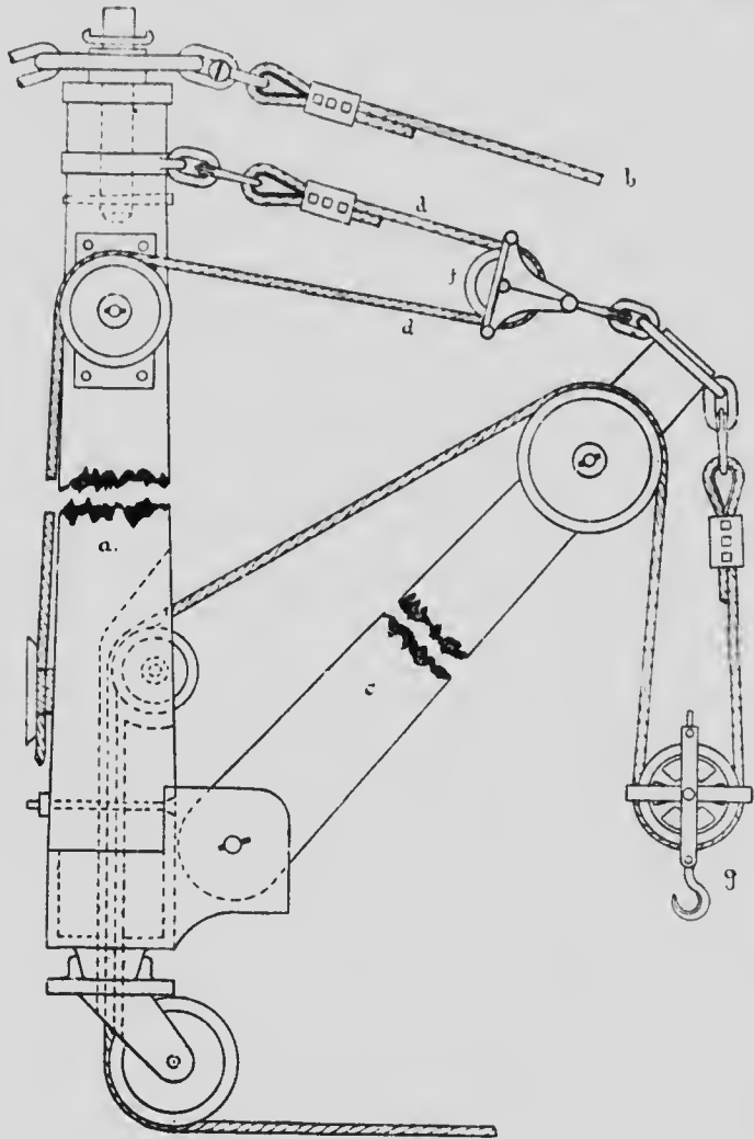
FIG. 9—Boom derrick.
