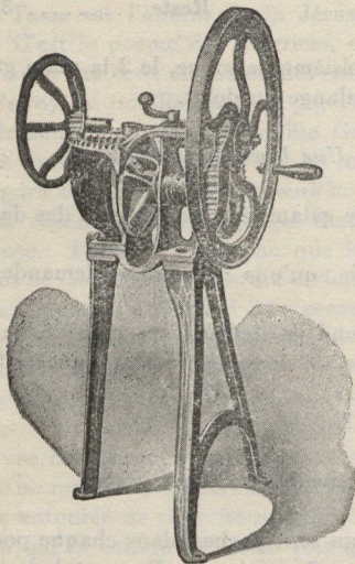
BROYEUR No. 1 — Capacité 1\frac{1}{4} lb. à la minute. Pesanteur 120 lbs. Prix $16.50.
