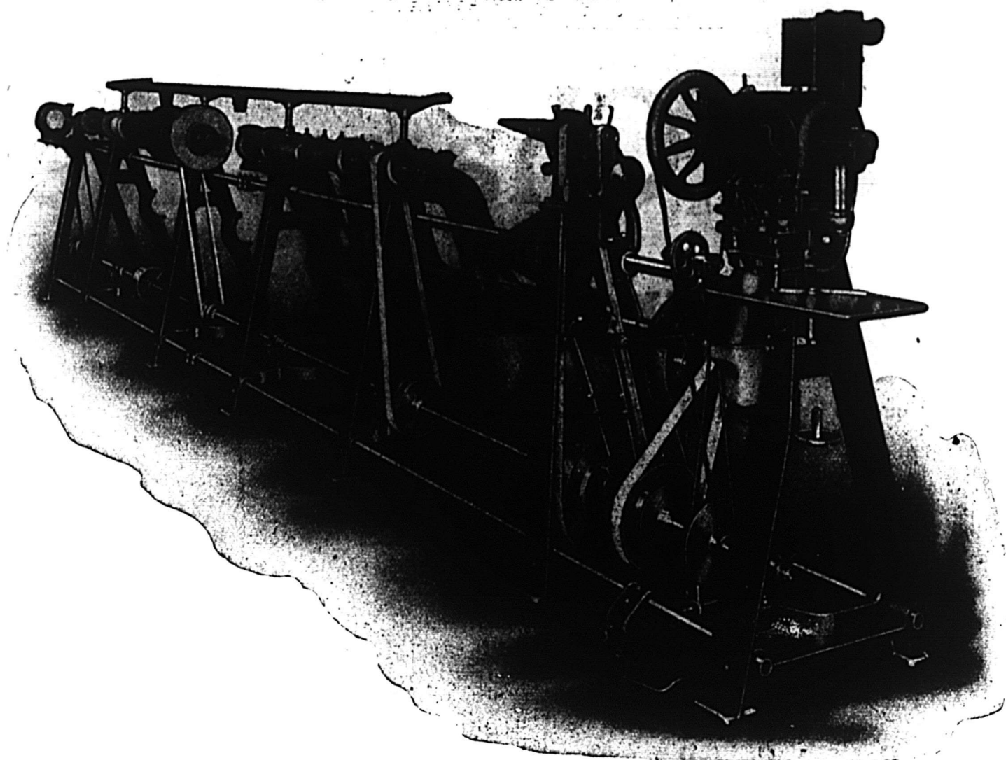
Installation Goodyear de 22 pieds pour réparations des chaussures, Modèle N
