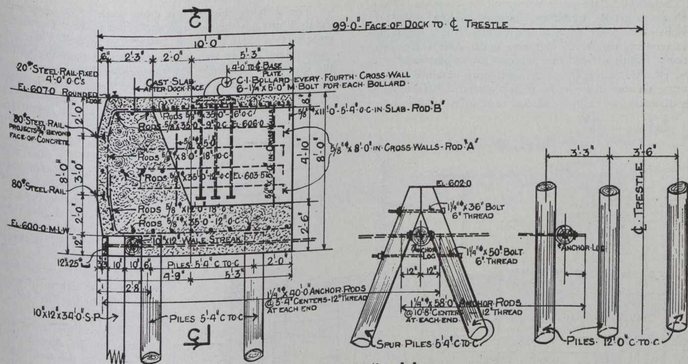
Fig. 4.—Section A A.
