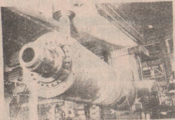
圖爲加工完畢的水泥磨筒體
