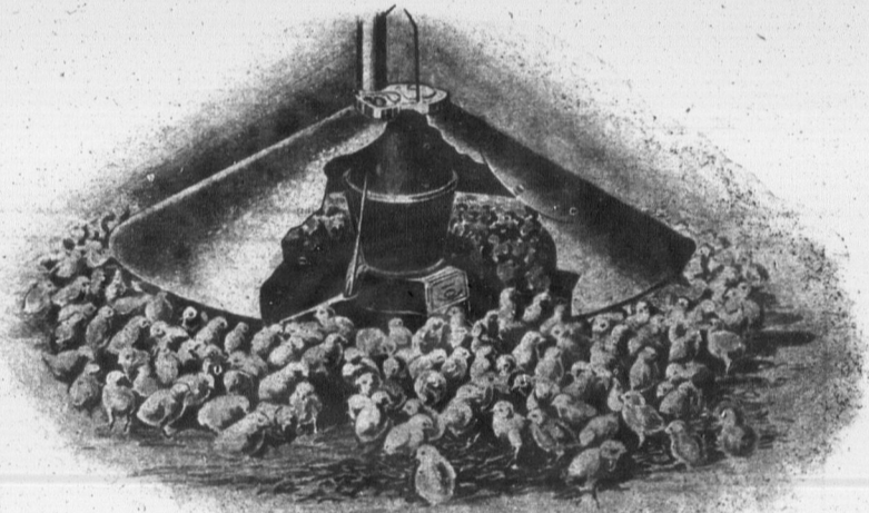
Poêle-éleveuse pour 400 poussins
