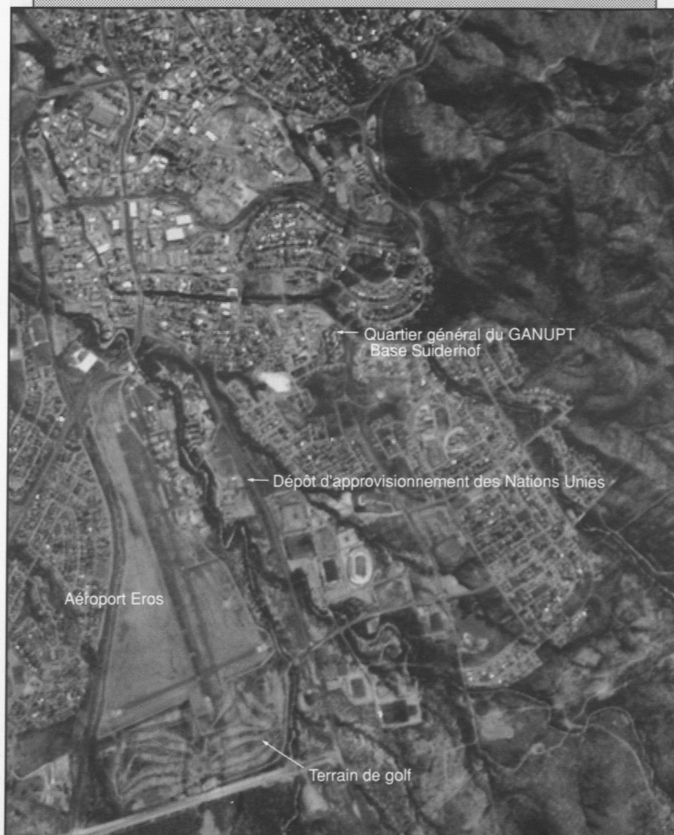
Figure 12 Image panchromatique de Windhoek, recueillie par le SPOT et montrant la zone où est installé le quartier général du GANUPT
