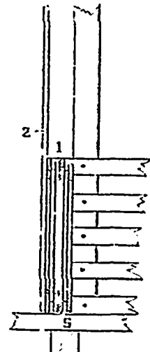
Fig. 5.—COUPE C. D. VUE DE CÔTÉ.
