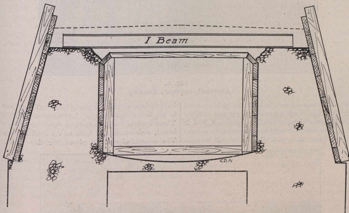
Fig. 6. Flat Top Culvert.
