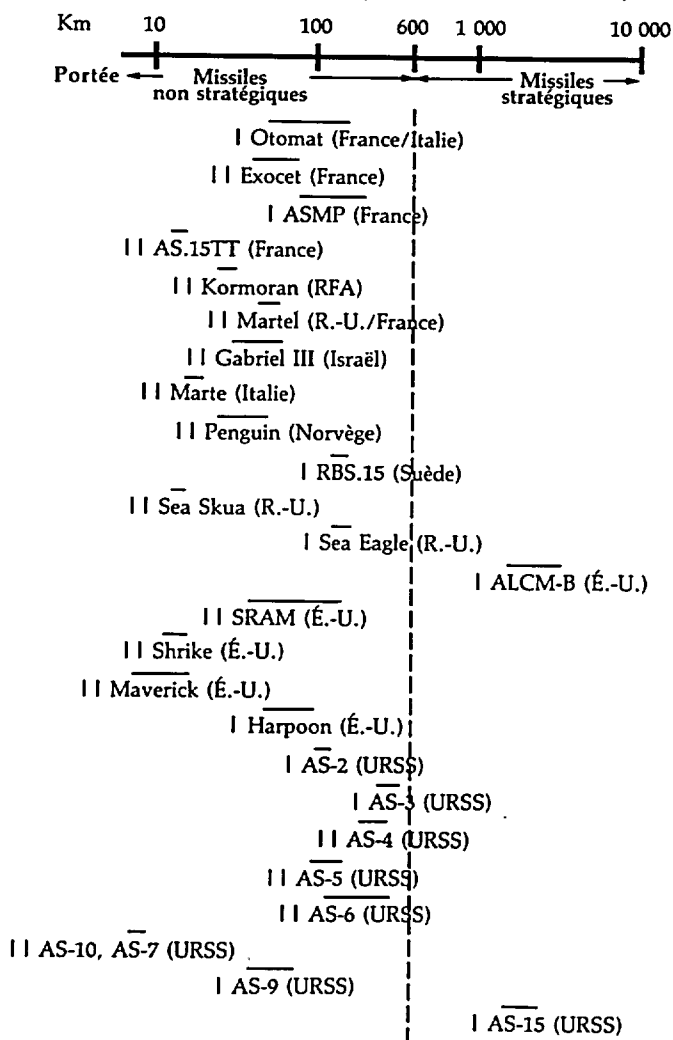
Figure 3 Missiles de croisière courants lancés à partir de l'air (selon le Jane's Weapon Systems , de 1987-1988)*
