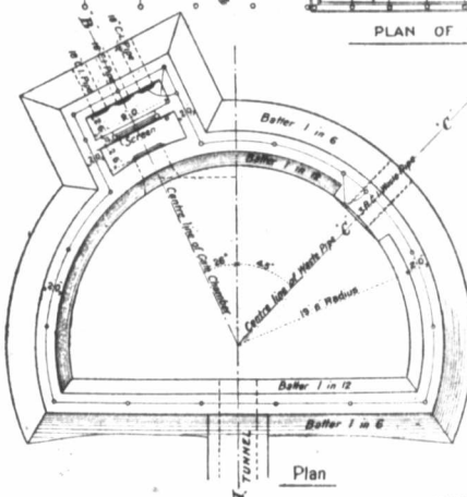
FOREBAY
