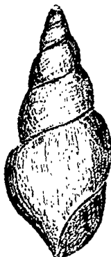
Fig. 190.— M. sulfusiformis (Hall).
