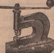
23—Fly Punch
