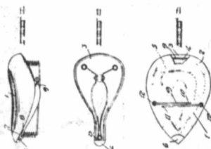
No. 132,358. Electric Frost Remover for Windows. Appareil électrique à enlever la gelée dans les fenêtres.
