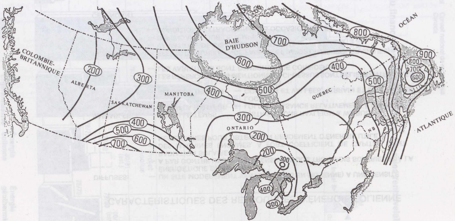
DENSITÉ ANNUELLE MOYENNE DE L'ÉNERGIE ÉOLIENNE À 50m D'ALTITUDE
