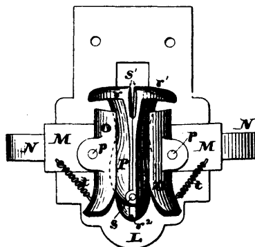
Coté's Heel Stiffener Machine.
