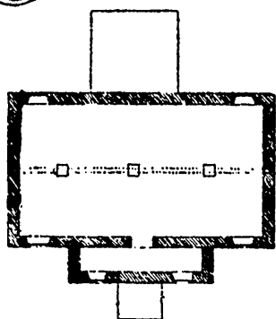
FONDATION
