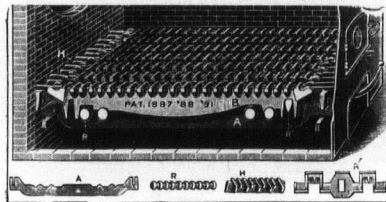
A. Hanger. B. Grate-Bar. H. Header. R. Roller. R'. Shaking Bar.
