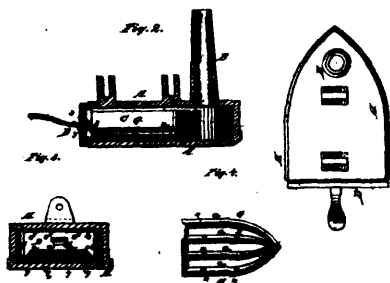
5295 Cottingham's Sad Iron.
