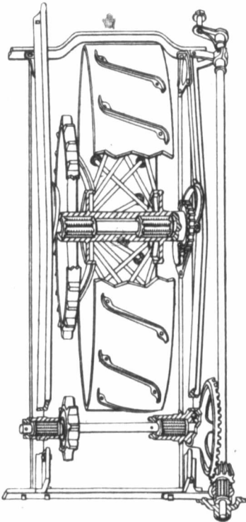
Fig. 17. Binder.
