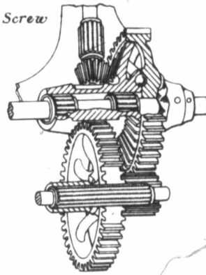
Fig. 18. Reaper.
