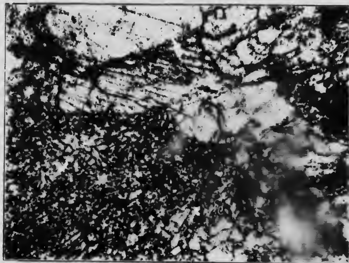
A. Microphotographie de roches de diopside-blanc grossièrement échantillonnées, lustrées naturellement, Montréal (Chrome Pit). (Page 28).
