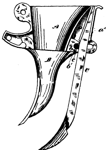
Galloway's Sowing Machine.
