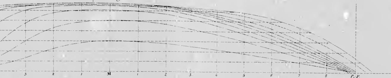
Fig 4. Plan des formes des Goëlettes des Pilotes du Saint-Laurent honorable Joseph Cauchon, hon David Price.
